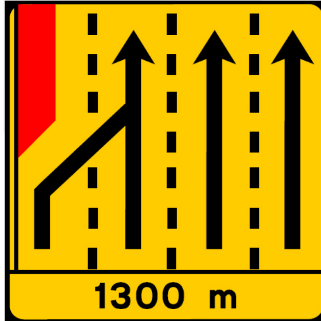
TD6 - Painel de estrangulamento à esquerda (4 vias) Desvio da via esquerda para a via central esquerda
